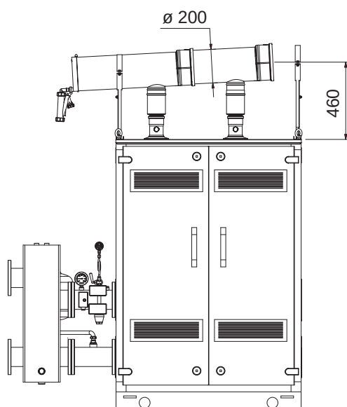
MURELLE EQUIPE 220 BOX ErP con kit colector humos cód. 8102530
