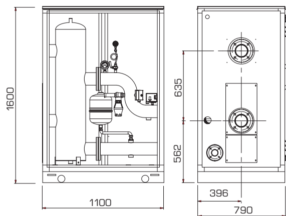
BOX DOBLE PARA SEPARADOR HIDRÁULICO Y TUBOS DE CONEXIÓN cód. 8101527 PARA "MURELLE EQUIPE 440-550 BOX ErP"
