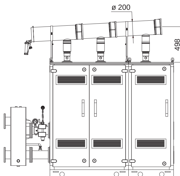
MURELLE EQUIPE 330 BOX ErP con kit colector humos cód. 8102531
