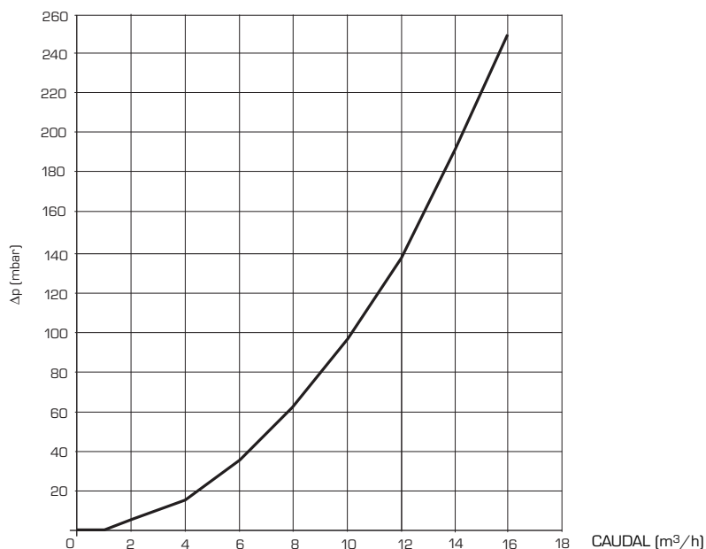
Separador hidraulico "DEWY EQUIPE 60-120-180-240 BOX"
