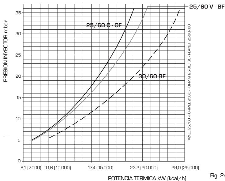
Diagrama presión/potencia para el gas propano (G31)
