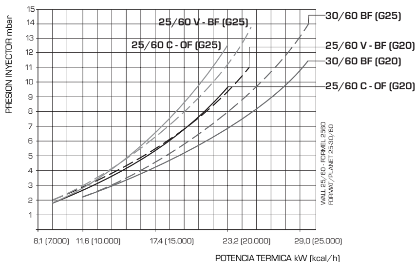
Diagrama presión/potencia para el gas natural (metano)
