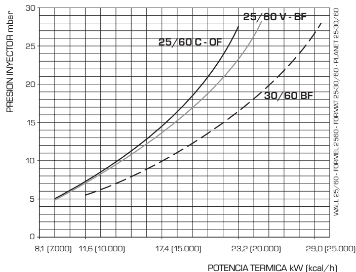
Diagrama presión/potencia para el gas butano (G30)
